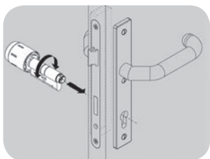
Fig. 18: Align cam
